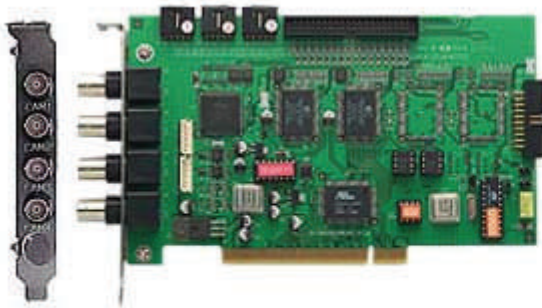
GV-650 BNC
